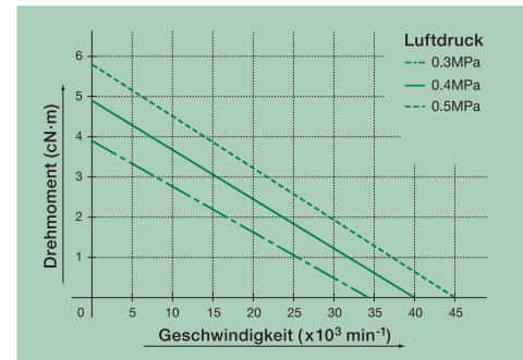
Drehmoment- und Leistungsdiagramm der SMS401 Serie
